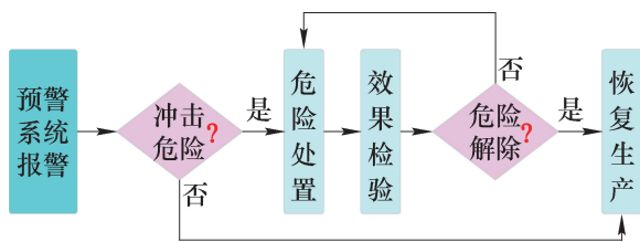
图 6 冲击危险处置流程
