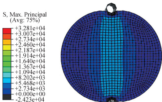
图3 弹性力学第一主应力云图
