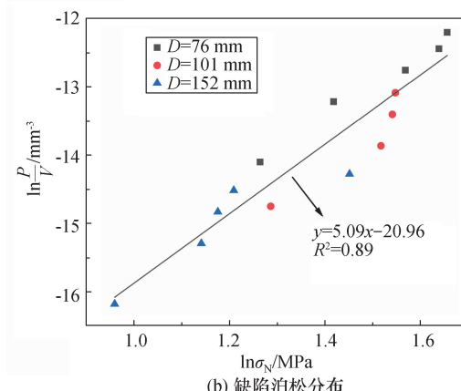
图5 2种缺陷分布下的拟合结果
