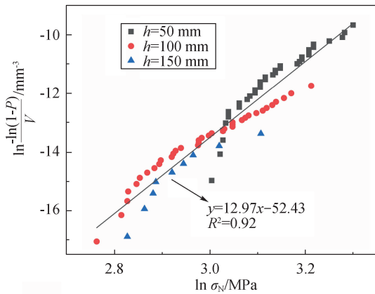
(a) 缺陷均匀分布
