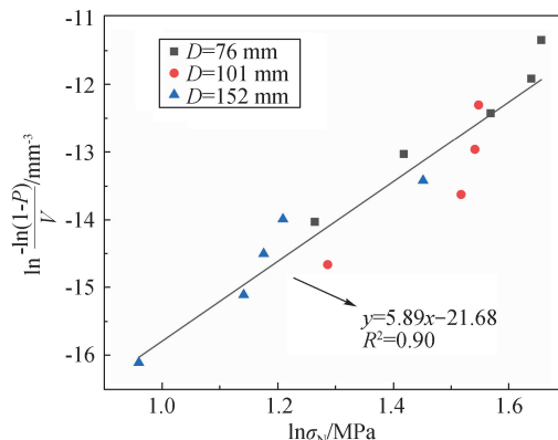
(a) 缺陷均匀分布
