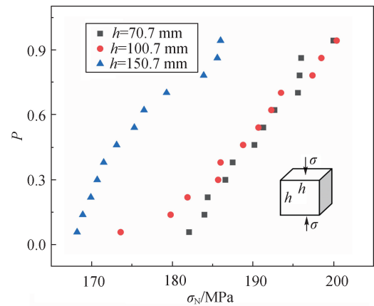
(a) 立方体单轴压缩经验概率
