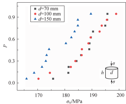
(b) 圆柱体单轴压缩经验概率
